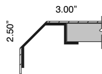
Bevel Edge Frame
