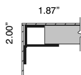
Square Edge Frame
